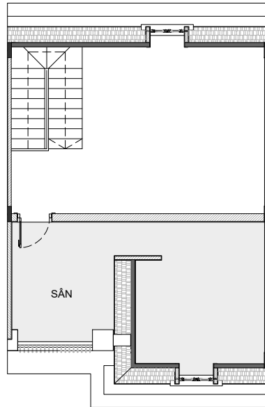
MẶT BẰNG TẦNG 5
